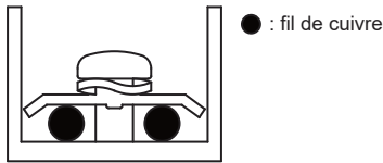
Connexions appropriées du câblage électrique
